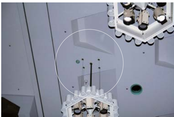
シャンデリア吊ワイヤーがガイド金具と接触
